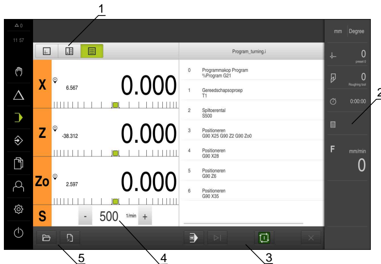
Afbeelding 16: Menu Programma-afloop
