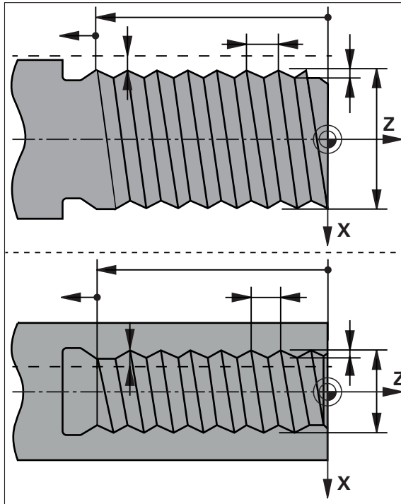
Afbeelding 46: Schematische weergave van de regel Schroefdraadsnijden (uitgebreid)
