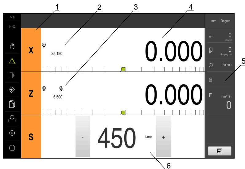
Afbeelding 15: Menu MDI-werkstand
