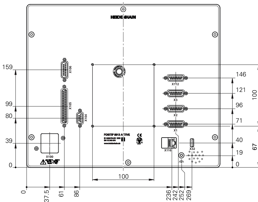
Afbeelding 53: Maatvoeringen van de achterzijde van het apparaat
