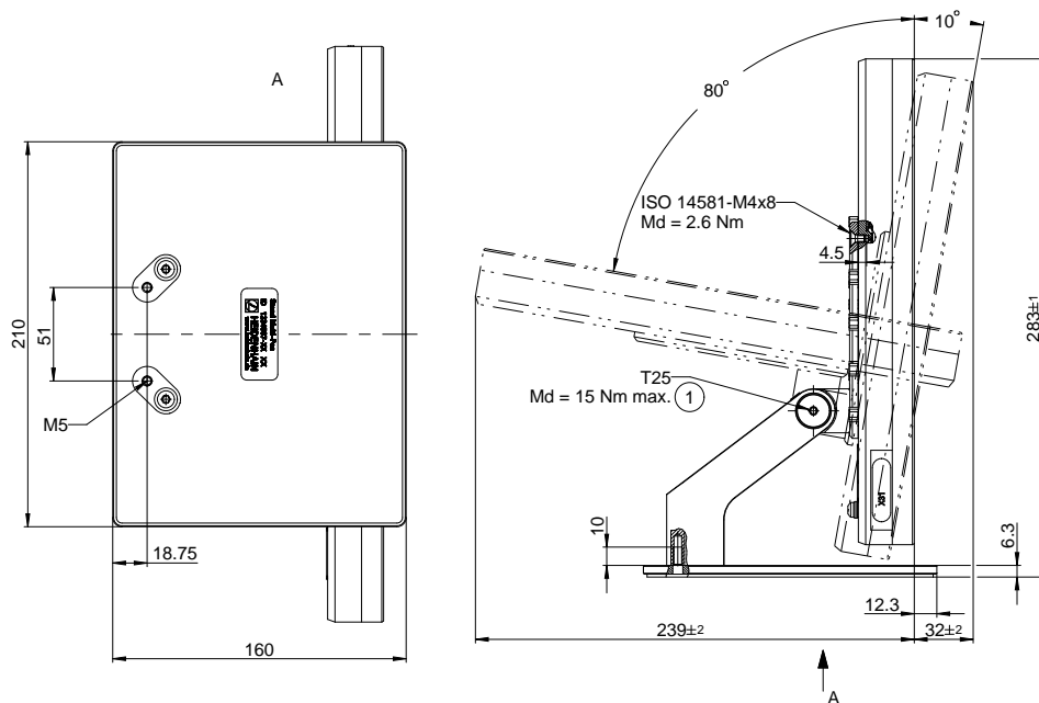
Afbeelding 58: Apparaatafmetingen met steunvoet Multi-Pos
