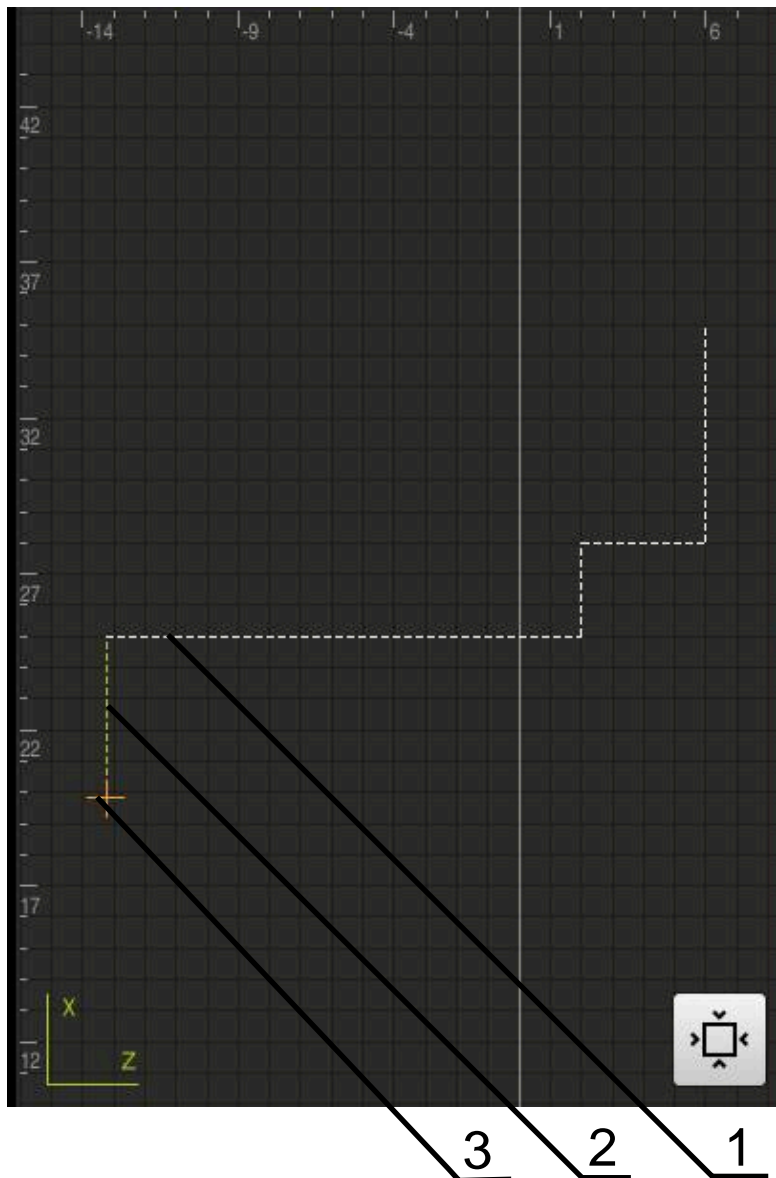
Afbeelding 38: Simulatievenster met contouraanzicht
