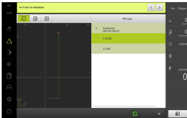
Afbeelding 41: Voorbeeld – uitvoering van een MDI-regel met schaalfactor
