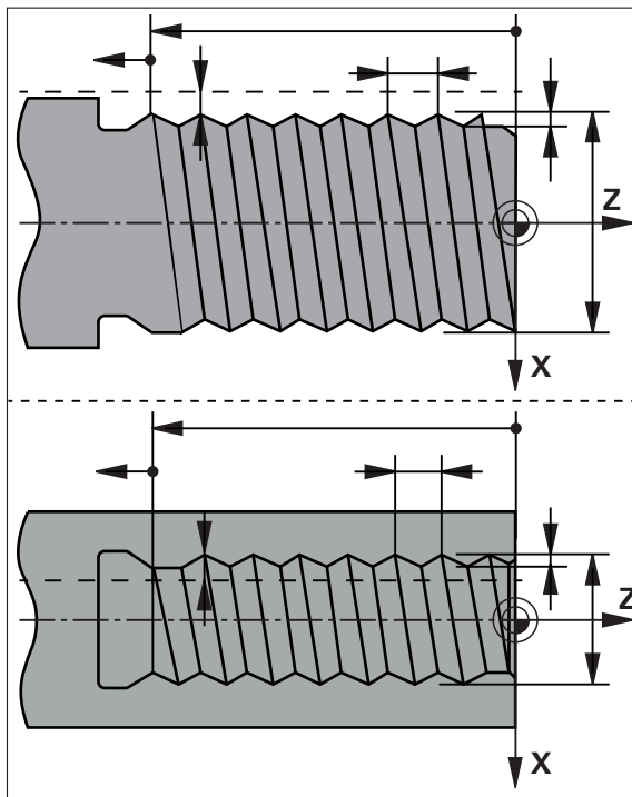
Afbeelding 36: Schematische weergave van de regel Schroefdraadsnijden (uitgebreid)
