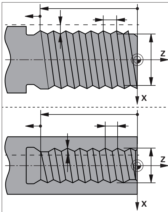
Afbeelding 35: Schematische weergave van de regel Schroefdraadsnijden (eenvoudig)
