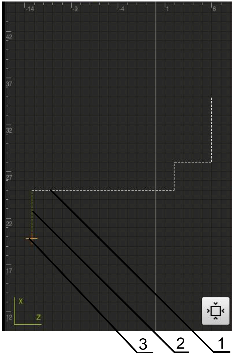
Afbeelding 48: Simulatievenster met contouraanzicht
