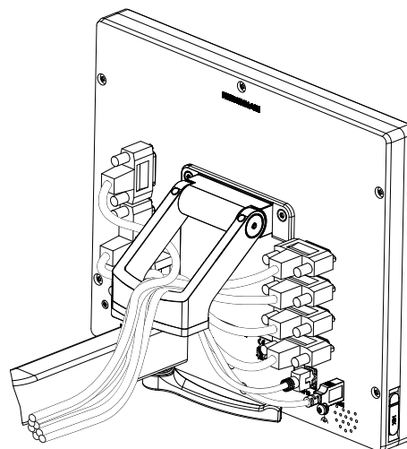
Afbeelding 9: Geleiden van de kabel op houder Multi-Pos
