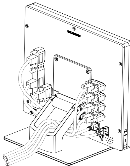
Afbeelding 7: Geleiden van de kabel op steunvoet Multi-Pos
