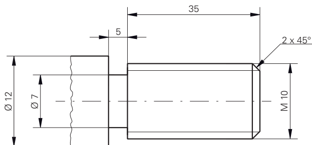
Afbeelding 26: Voorbeeldwerkstuk – technische tekening
