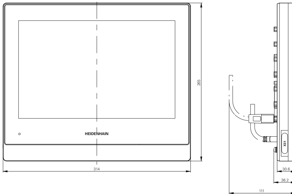
Afbeelding 52: Maatvoeringen van de behuizing
