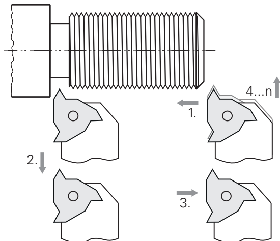
Afbeelding 30: Voorbeeldwerkstuk – Schroefdraad maken
