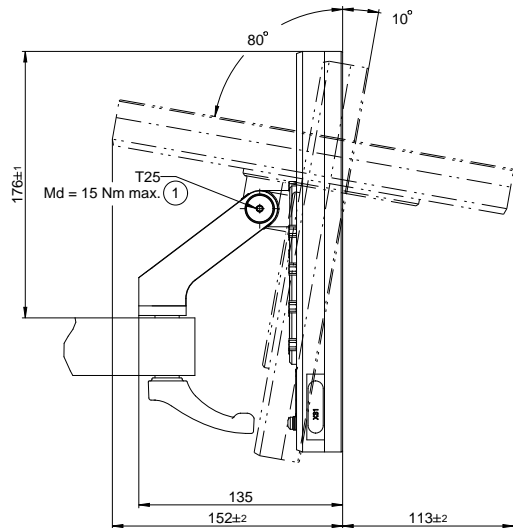
Afbeelding 59: Apparaatafmetingen met houder Multi-Pos
