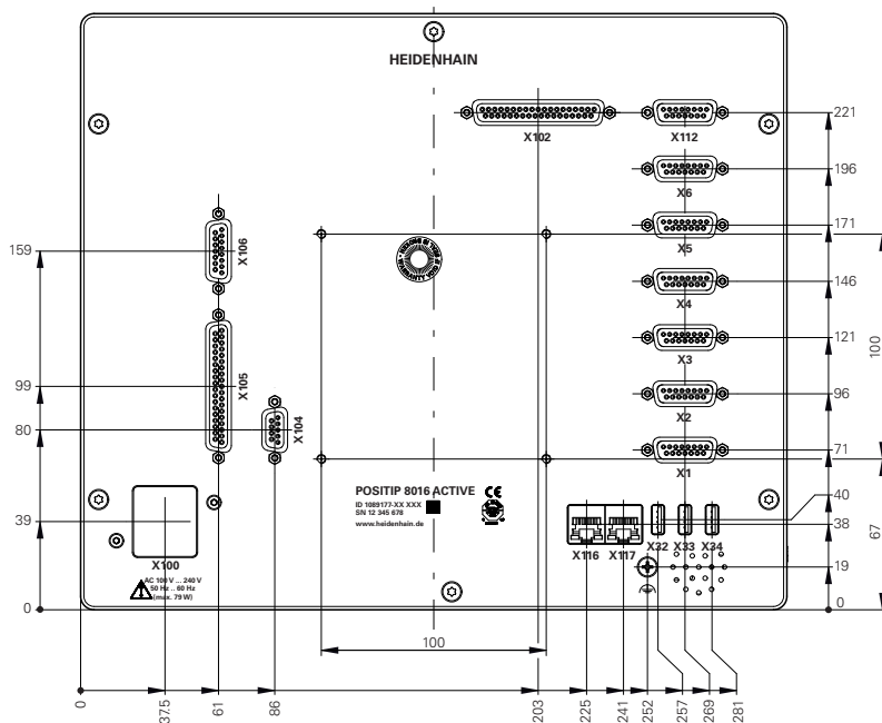
Afbeelding 55: Maatvoeringen van de achterzijde van het apparaat van de apparaten met ID 1089177-xx
