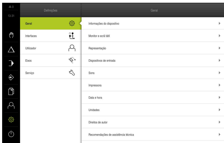
Figura 14: Menu Definições
