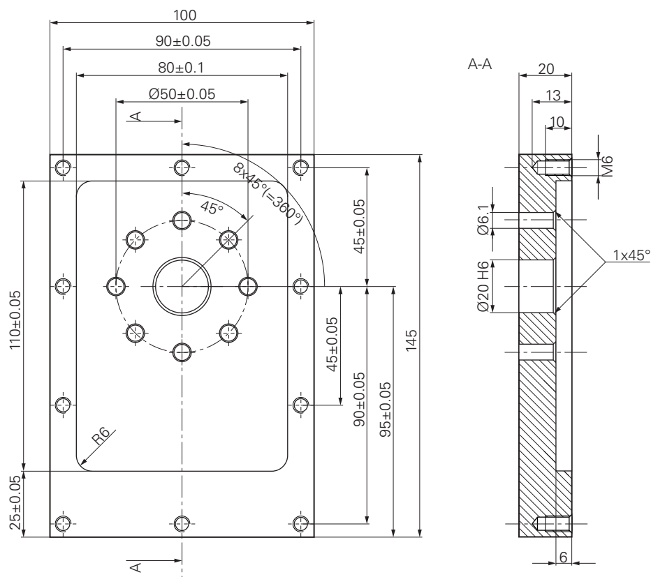
Illustration 16 : Exemple de pièce – Dessin technique
