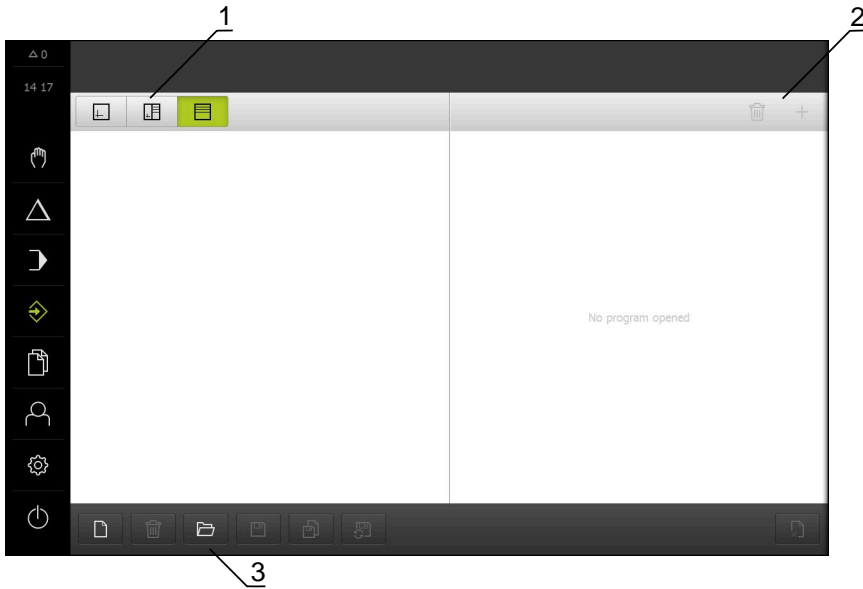
Şekil 9: Programlama menüsü
