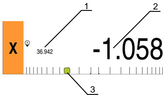
Figura 46: Vista Percurso restante com posição com ajuda gráfica ao posicionamento
