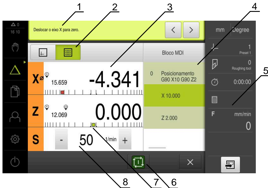
Figura 44: Exemplo de bloco no modo de funcionamento MDI
