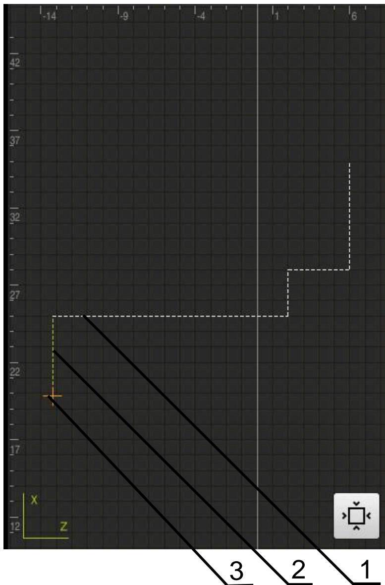
Figura 45: Janela de simulação com vista de contorno
