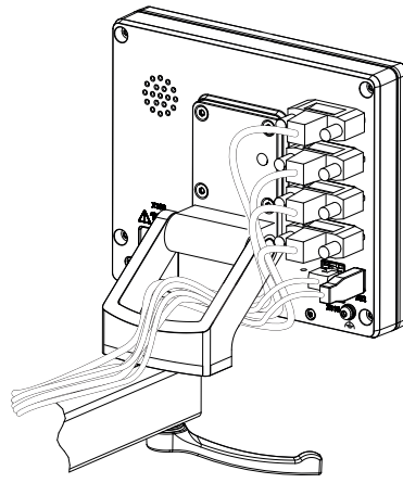
Şekil 22: Multi-Pos tutucudaki kablo yönlendirmesi
