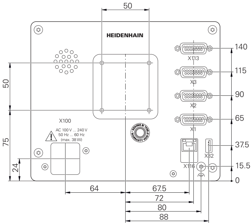
Şekil 34: 1089178-xx ünitelerinin ve arka boyutları
