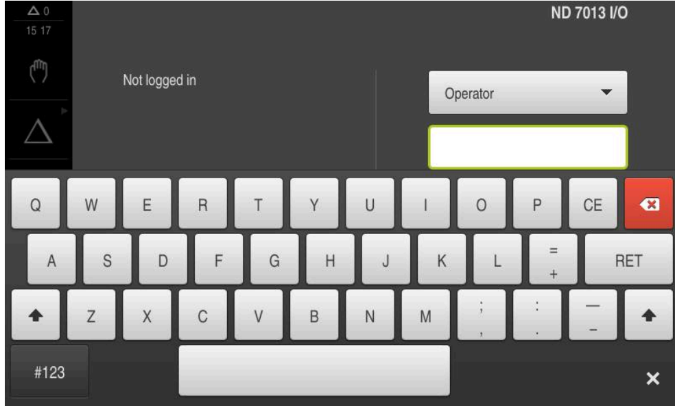
Şekil 1: Ekran klavyesi
