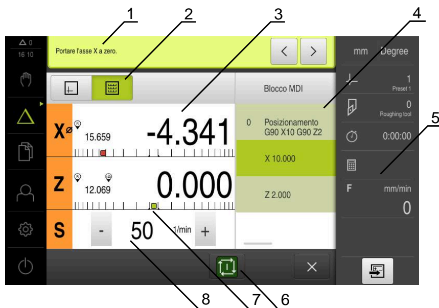
Figura 44: Esempio di blocco in modalità MDI
