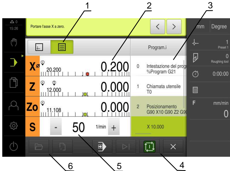
Figura 49: Esempio di programma in modalità Esecuzione programma
