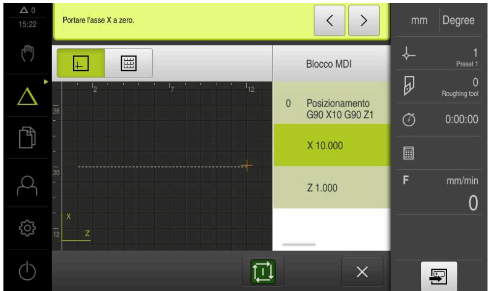
Figura 47: esempio – blocco MDI
