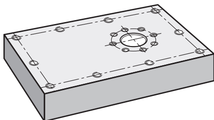
Kuva 20: Esimerkkityökappale – Reikärievin valmistus
