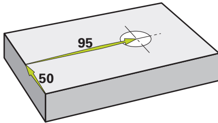
Şekil 15: Örnek malzeme – Geçiş deliğinin oluşturulması
