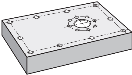
Şekil 20: Örnek malzeme – Delik sırasının oluşturulması
