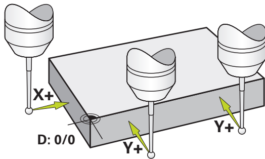
Şekil 14: Örnek malzeme – Referans noktasının belirlenmesi
