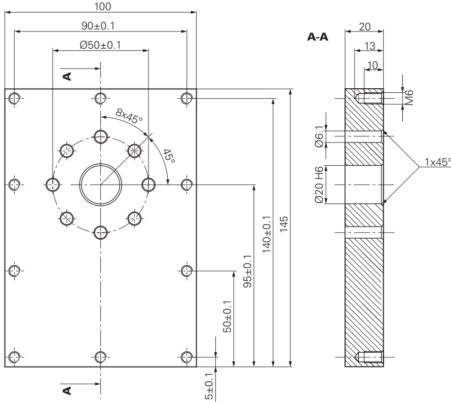
Şekil 13: Örnek malzeme – Teknik çizim
