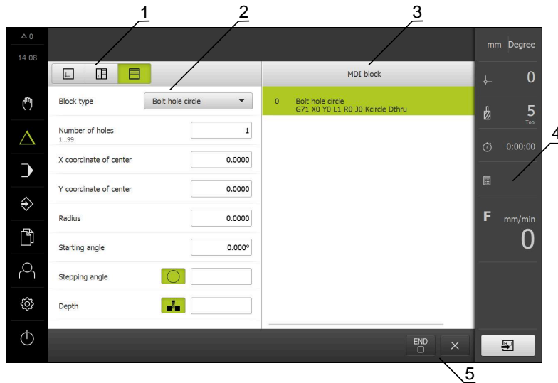
Kuva 7: Valintaikkuna MDI-lause
