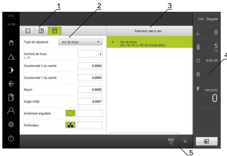
Figure 7 : Dialogue Exécution pas à pas
