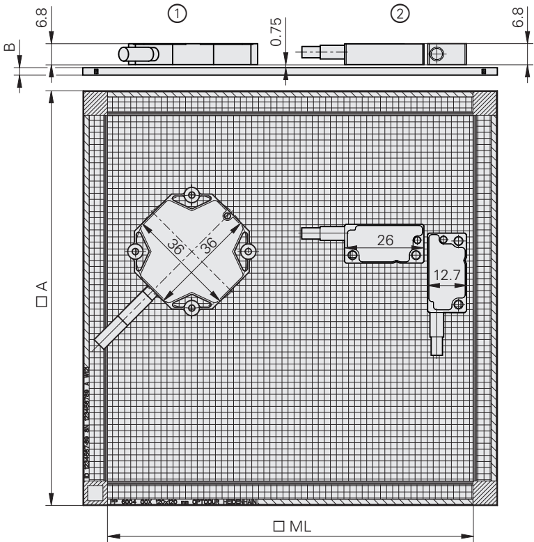
Umlaufende Referenzmarke
