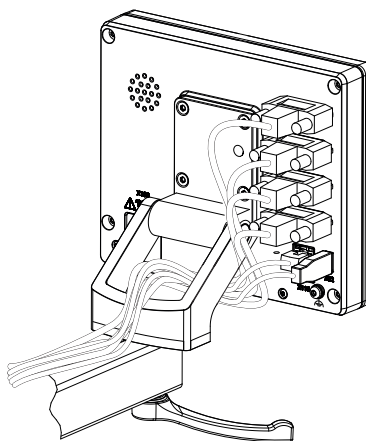
Figura 22: Passagem dos cabos no suporte Multi-Pos
