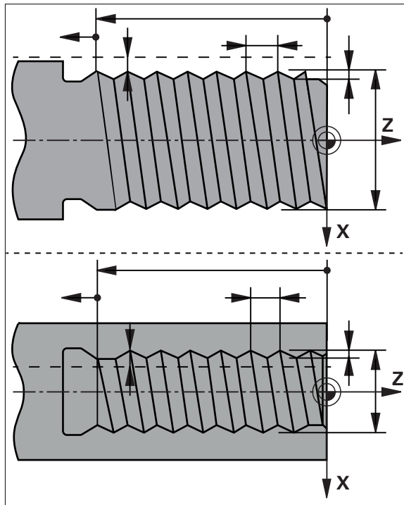
Figura 45: Representação esquemática do bloco Roscagem à lâmina (avançada)
