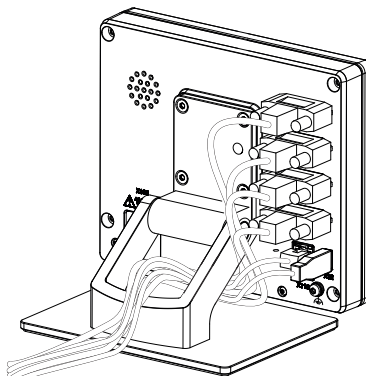
Figura 20: Passagem dos cabos no pedestal Multi-Pos
