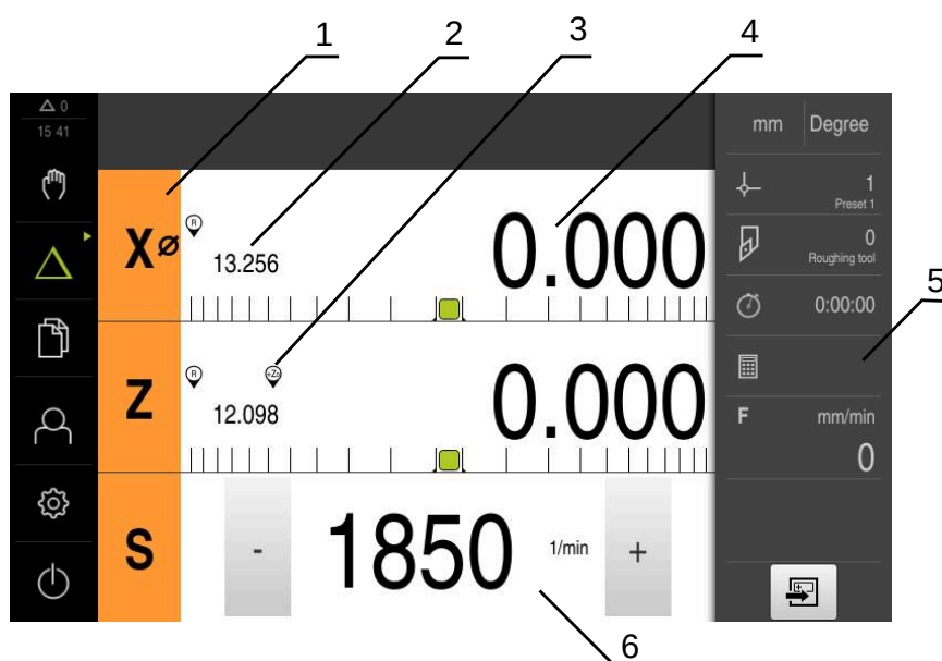
Figura 4: Menu Modo de funcionamento MDI
