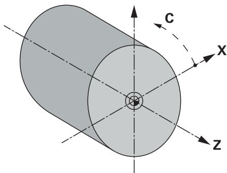
Figura 25: Correspondência do sistema de coordenadas retangulares com a peça de trabalho
