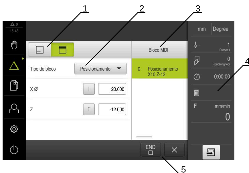
Figura 5: Diálogo Bloco MDI
