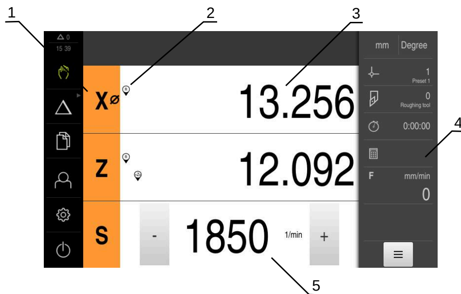
Figura 3: Menu Modo manual
