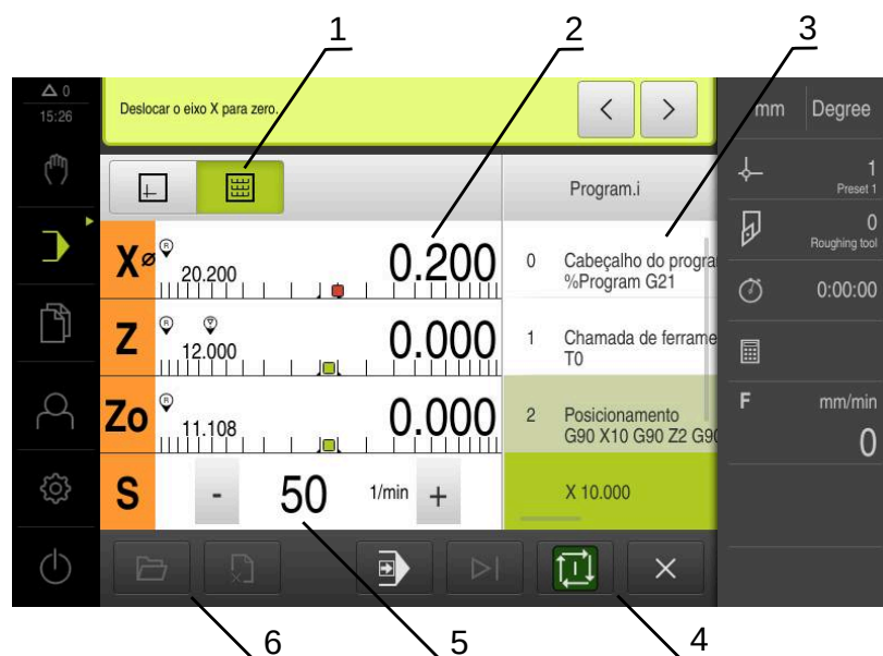
Figura 51: Exemplo de programa no modo de funcionamento Execução do programa
