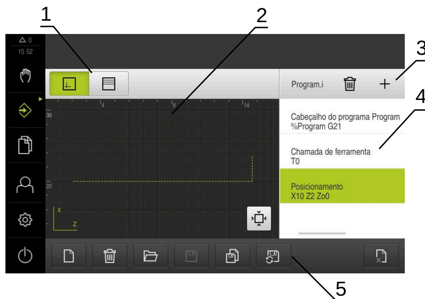
Figura 8: Menu Programação com a janela de simulação aberta
