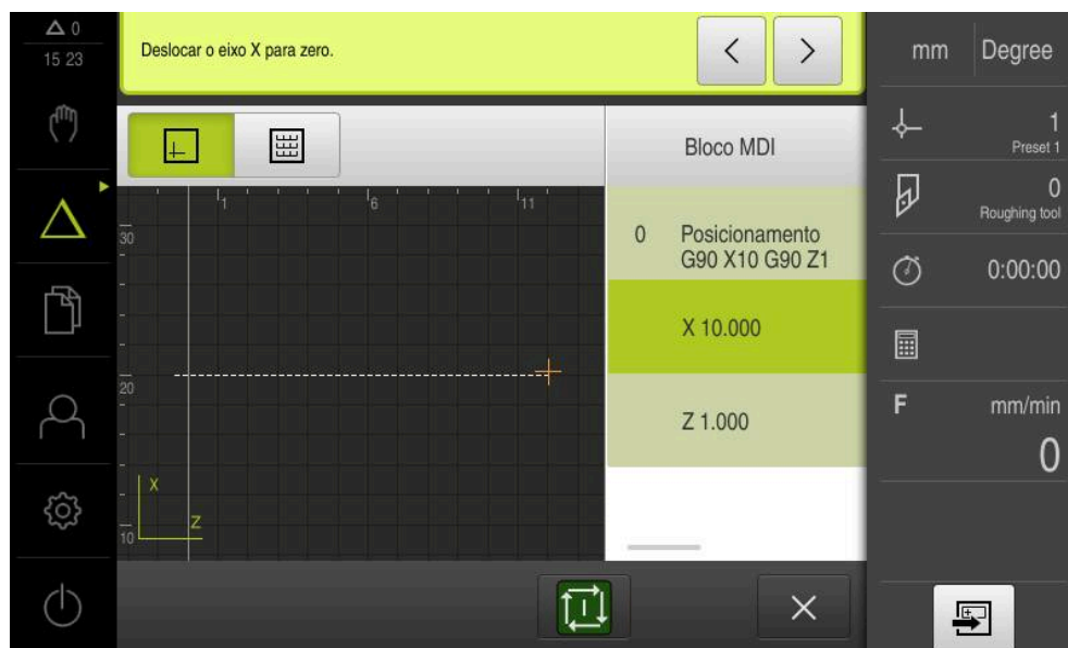
Figura 50: Exemplo – Execução de um bloco MDI com fator de escala
