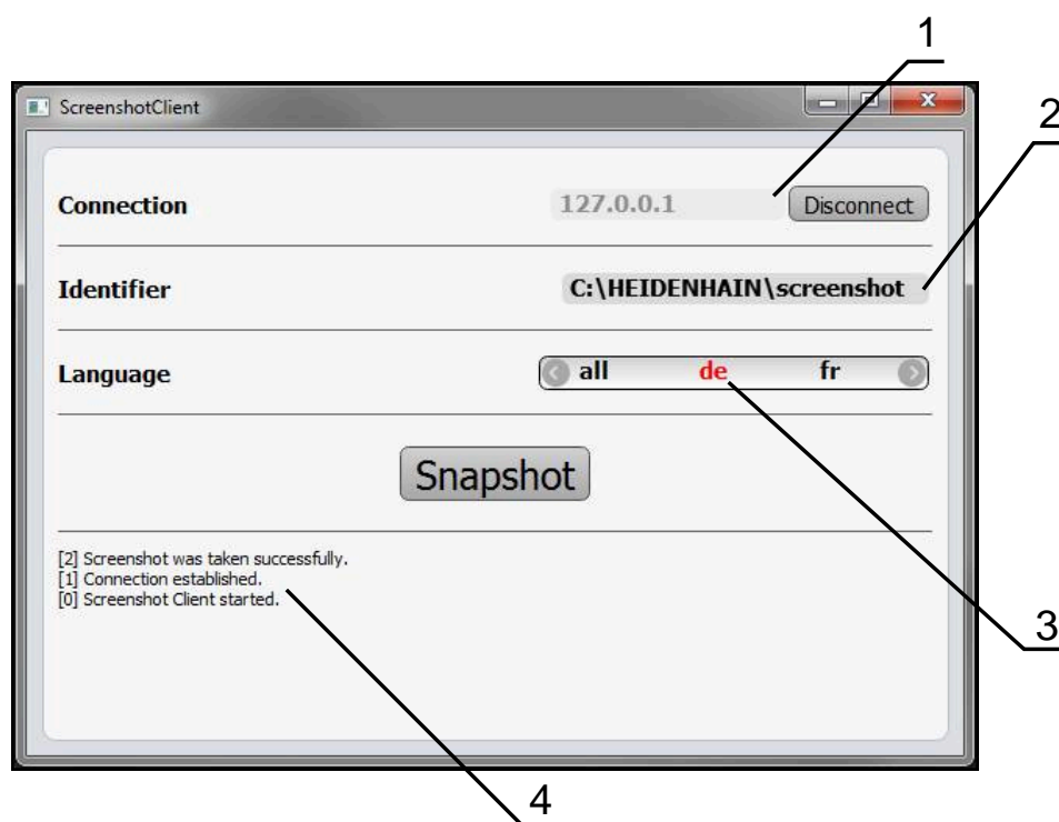
Afbeelding 20: Gebruikersinterface van ScreenshotClient
