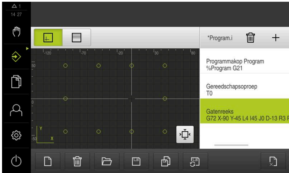
Afbeelding 18: Voorbeeldwerkstuk - simulatievenster
