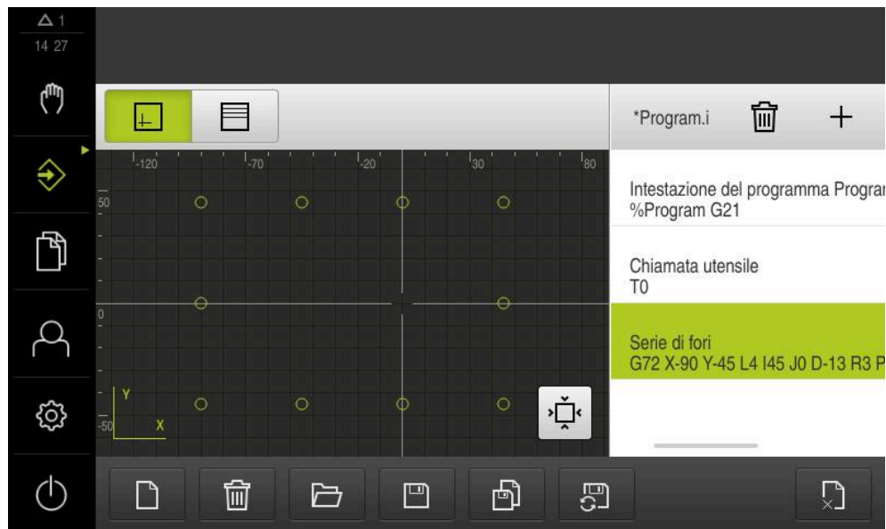
Figura 19: pezzo esemplificativo - finestra di simulazione
