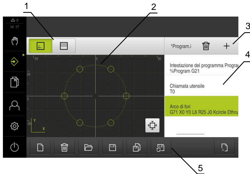
Figura 7: Menu Programmazione con finestra di simulazione aperta
