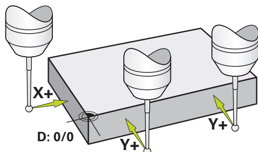
Figura 14: pezzo esemplificativo – definizione origine
