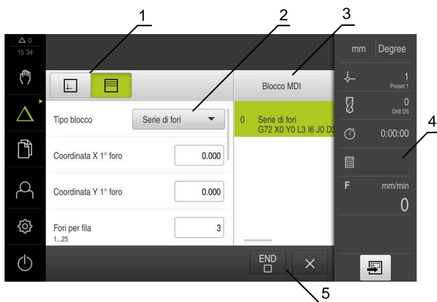
Figura 4: Dialogo Blocco MDI
