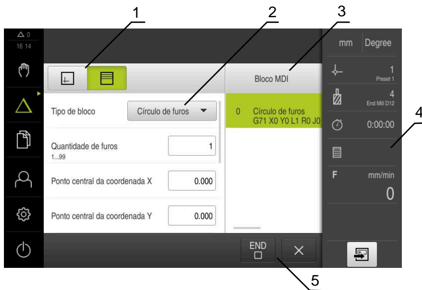
Figura 7: Diálogo Bloco MDI
