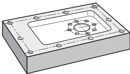
Kuva 25: Esimerkkityökappale – Reikäriivin valmistus
