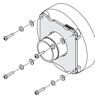
Anbau Abtasteinheit
