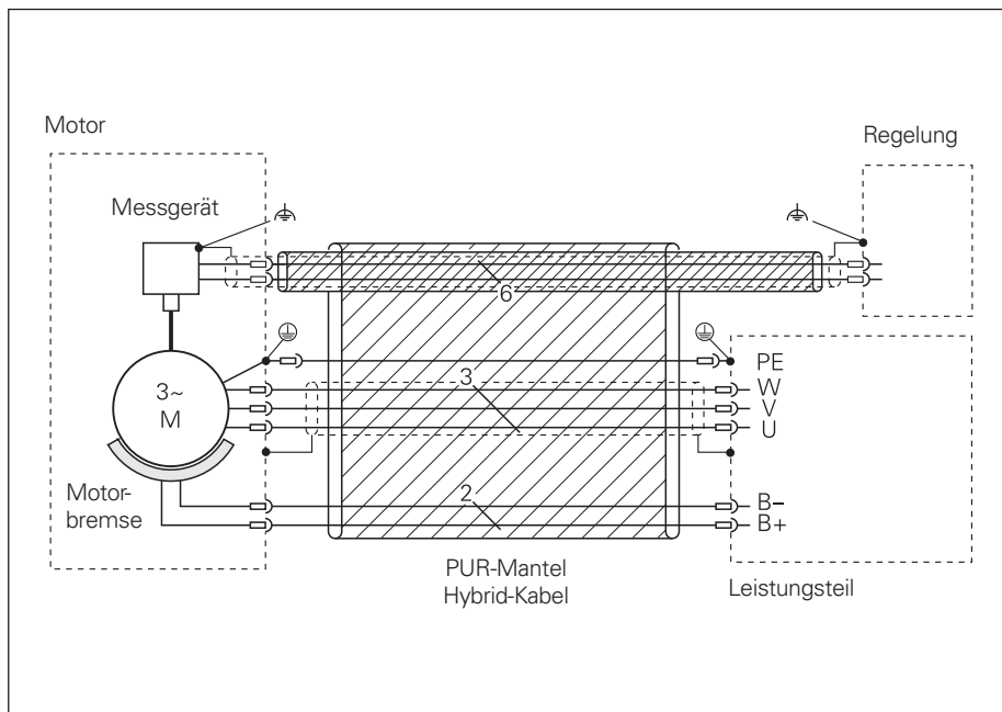
Erdungsplan
