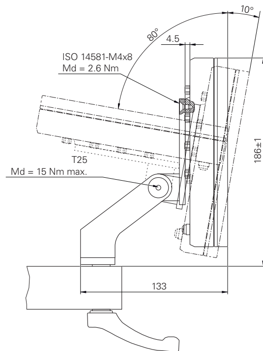
圖形 35: 含多位置固定架的產品尺寸
