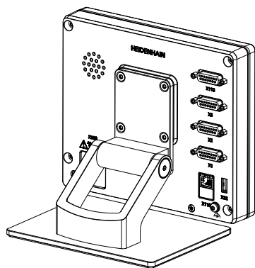
Figura 15: apparecchiatura montata su base di supporto Multi-Pos
