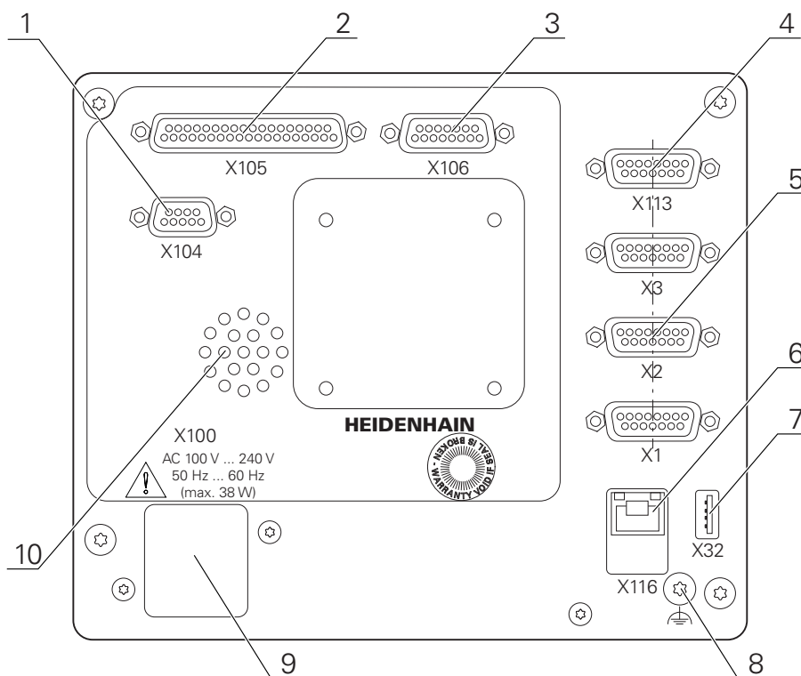
Figura 20: Retro per apparecchiature con ID 1089182-01
