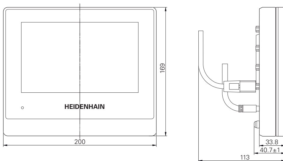
Figura 28: Dimensioni del corpo delle apparecchiature con ID 1089181-xx
