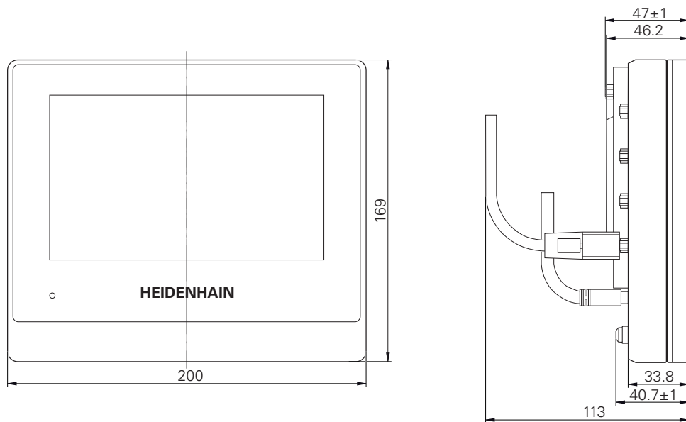
Figura 29: Dimensioni del corpo delle apparecchiature con ID 1089182-xx
