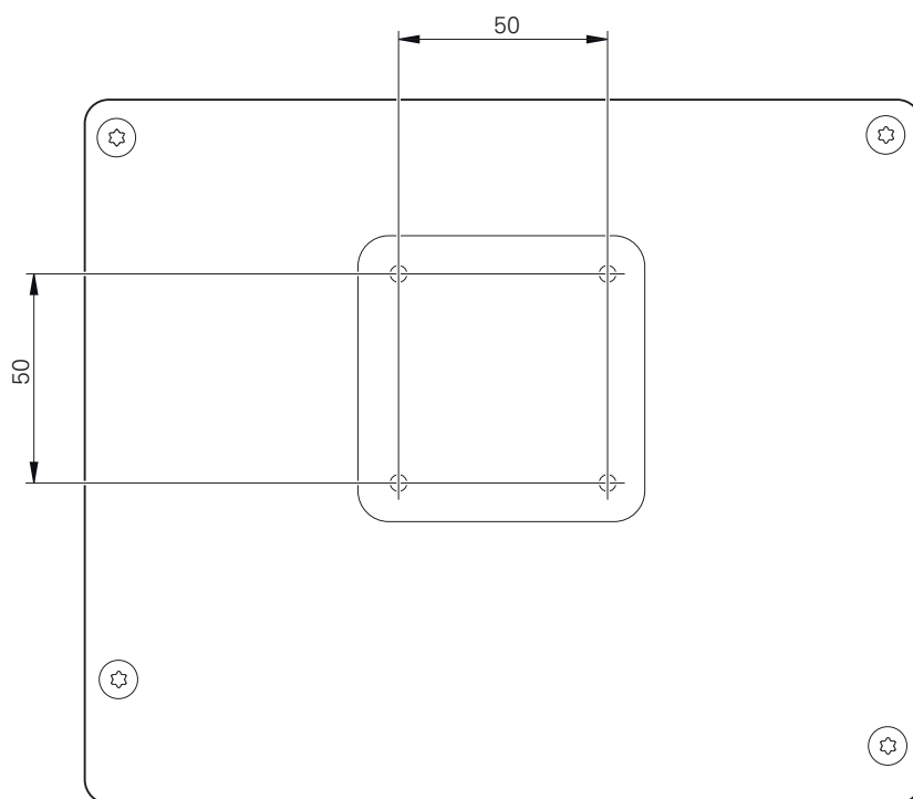
Figura 10: Quotatura del retro dell'apparecchiatura
