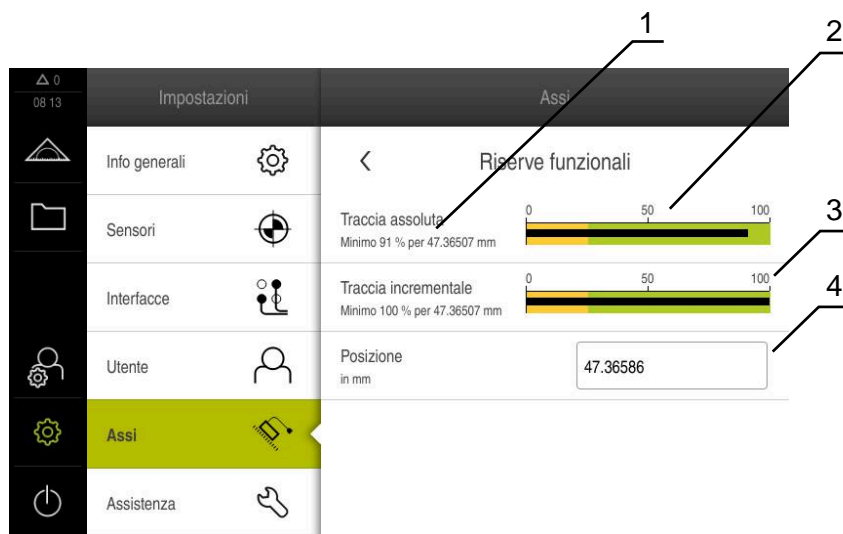
Figura 27: Esempio di riserve funzionali di un tastatore di misura
