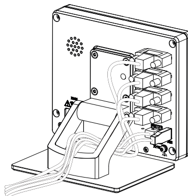
Figura 16: passaggio dei cavi con base di supporto Multi-Pos
