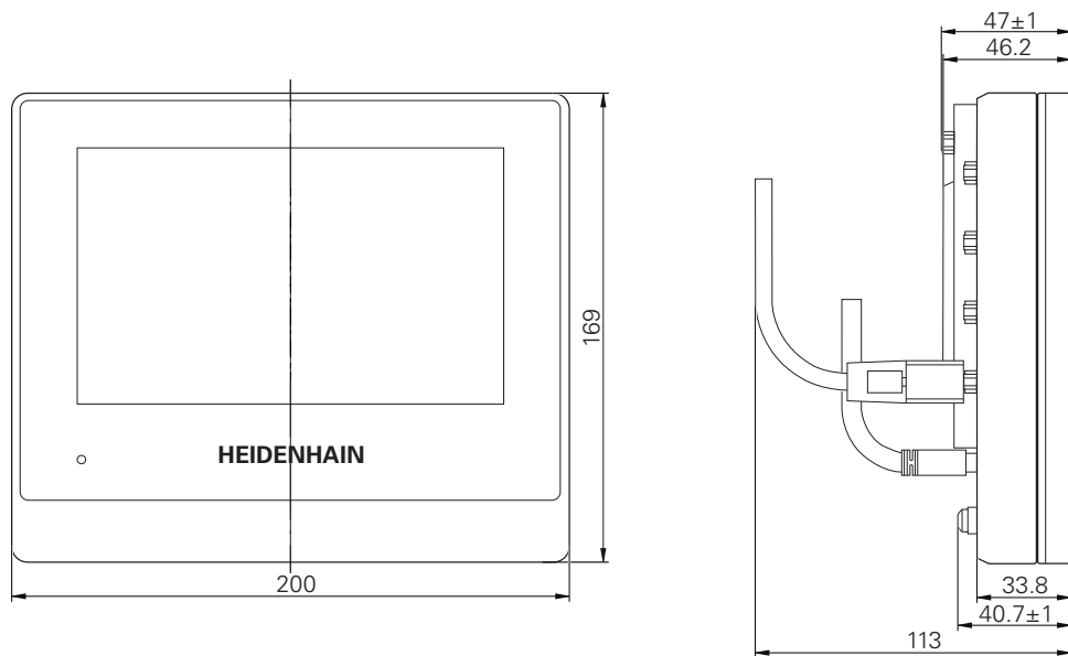
圖形 29: 具有ID 1089182-xx的裝置之外殼尺寸
