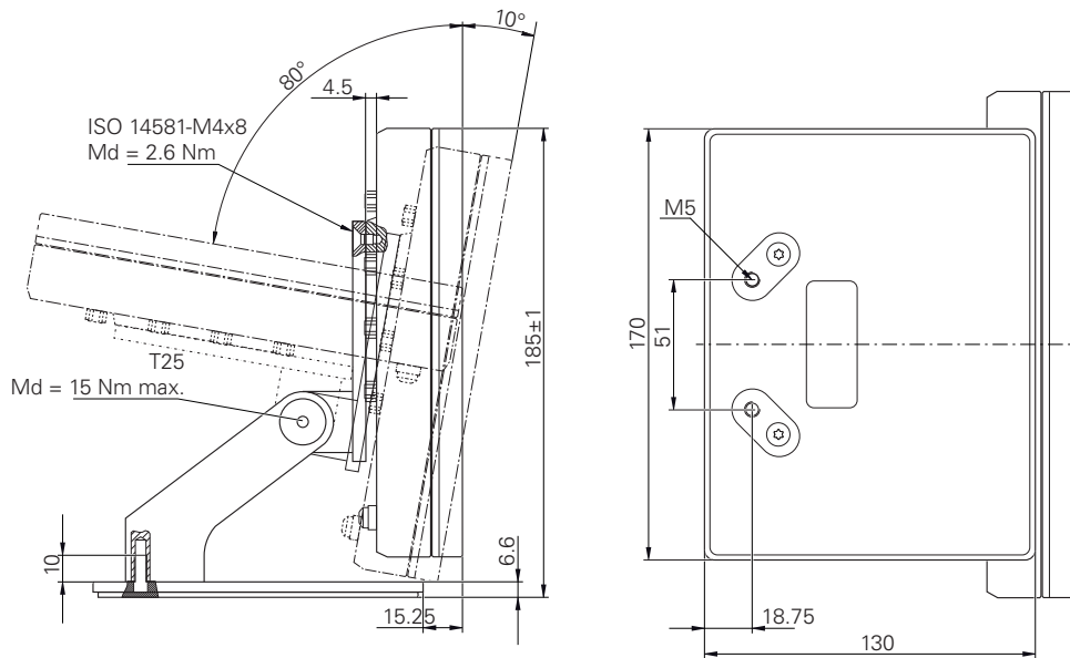
圖形 34: 含多位置立架的產品尺寸
