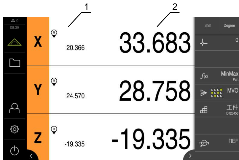
圖形 37: 量測功能表含接觸式探針
