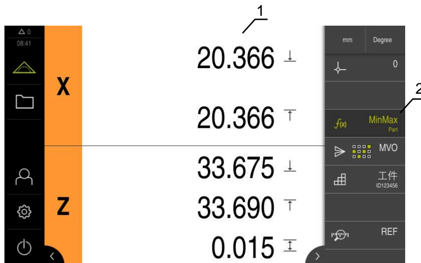
圖形 39: 量測功能表含啟動的MinMax功能
