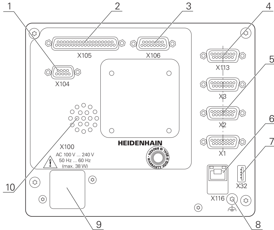
圖形 20: 1089182-xx的裝置背板
