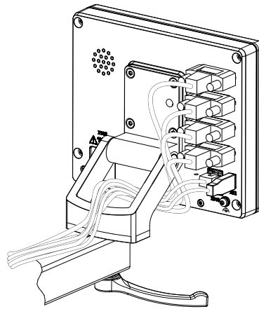
圖形 18: 多位置固定架上的纜線佈線
