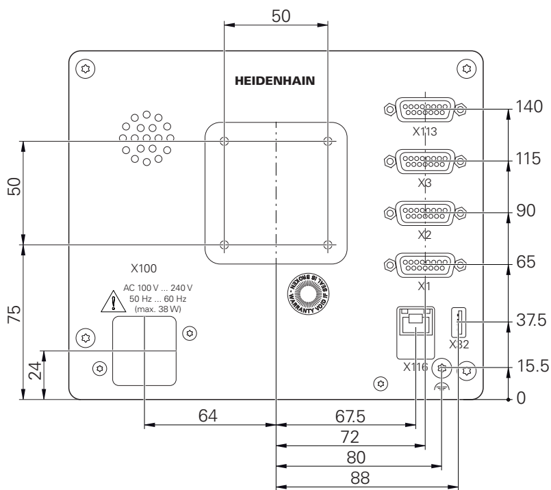
圖形 30: 具有ID 1089181-xx的裝置之後面板尺寸
