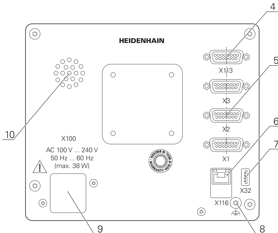
圖形 19: ID 1089181-01的裝置背板
