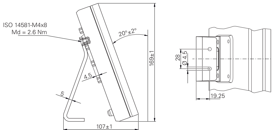
圖形 32: 含單位置立架的產品尺寸
