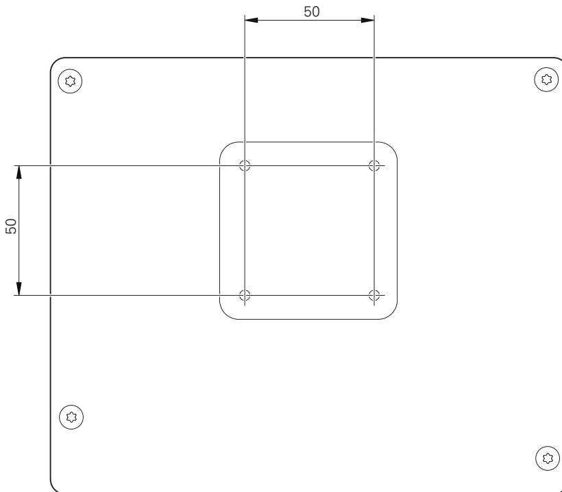
圖形 10: 產品背板的尺寸
