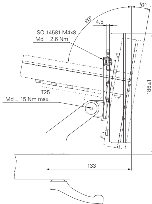
圖形 35: 含多位置固定架的產品尺寸
