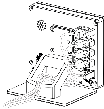
圖形 16: 多位置立架上的纜線佈線
