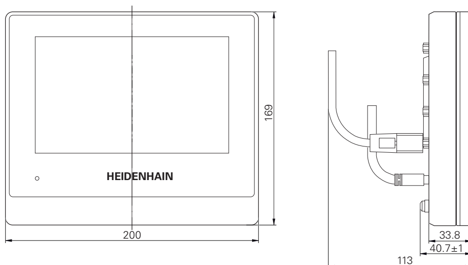
圖形 28: 具有ID 1089181-xx的裝置之外殼尺寸
