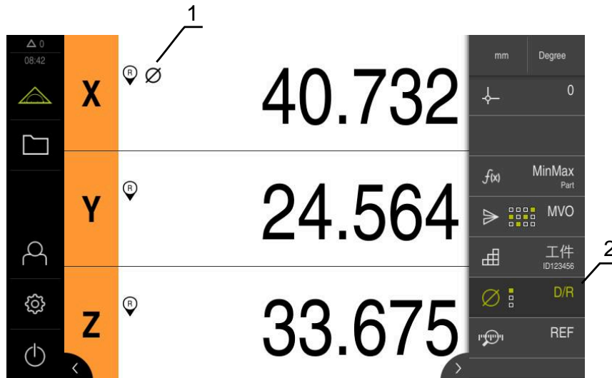
圖形 40: 量測功能表含啟動的D/R功能
