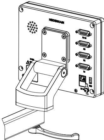
圖形 17: 產品固接在多位置固定架上
