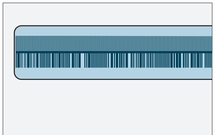
Schematische Darstellung einer Codestruktur mit zusätzlicher Inkrementalspur (Beispiel für LC 485)
