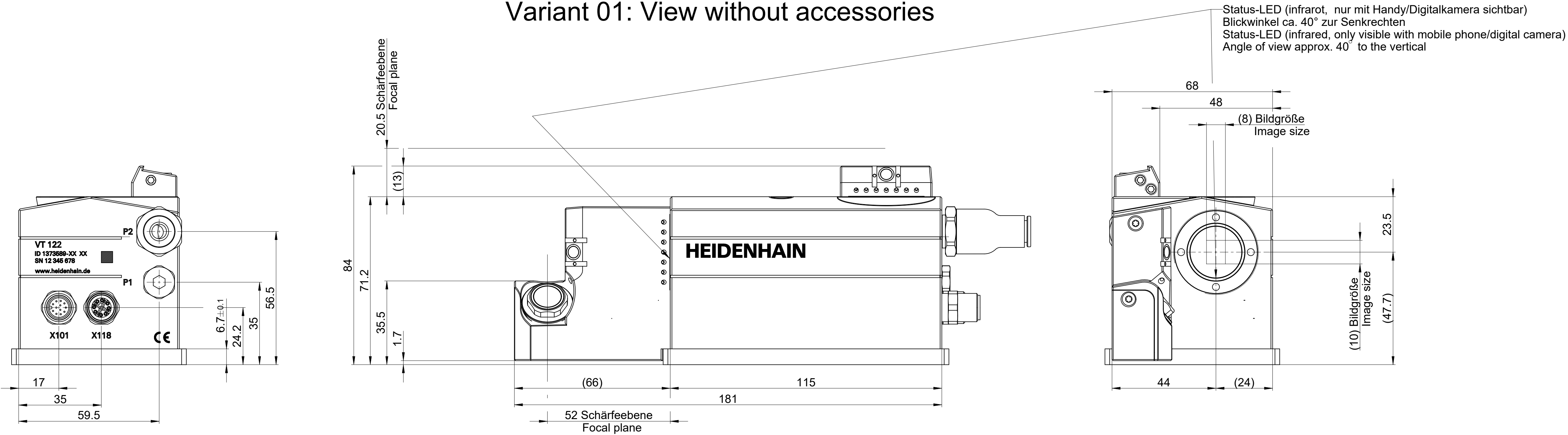
Variante 01: Ansicht ohne Zubehör Variant 01: View without accessories
