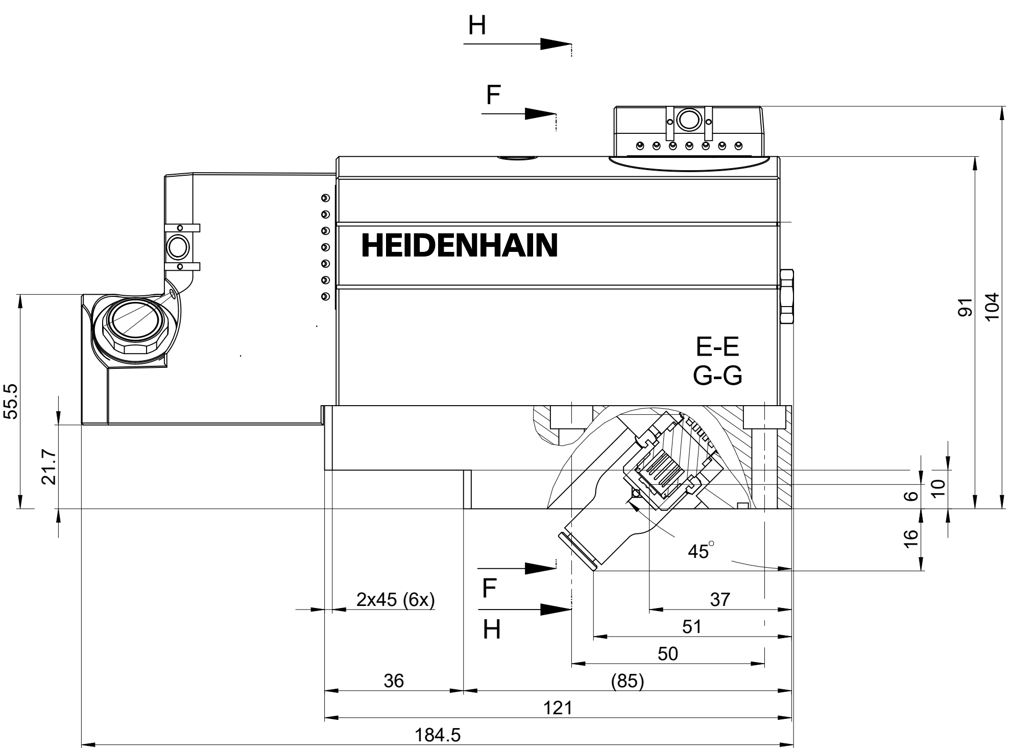
Variante 02: Ansicht ohne Zubehör Variant 02: View without accessories
