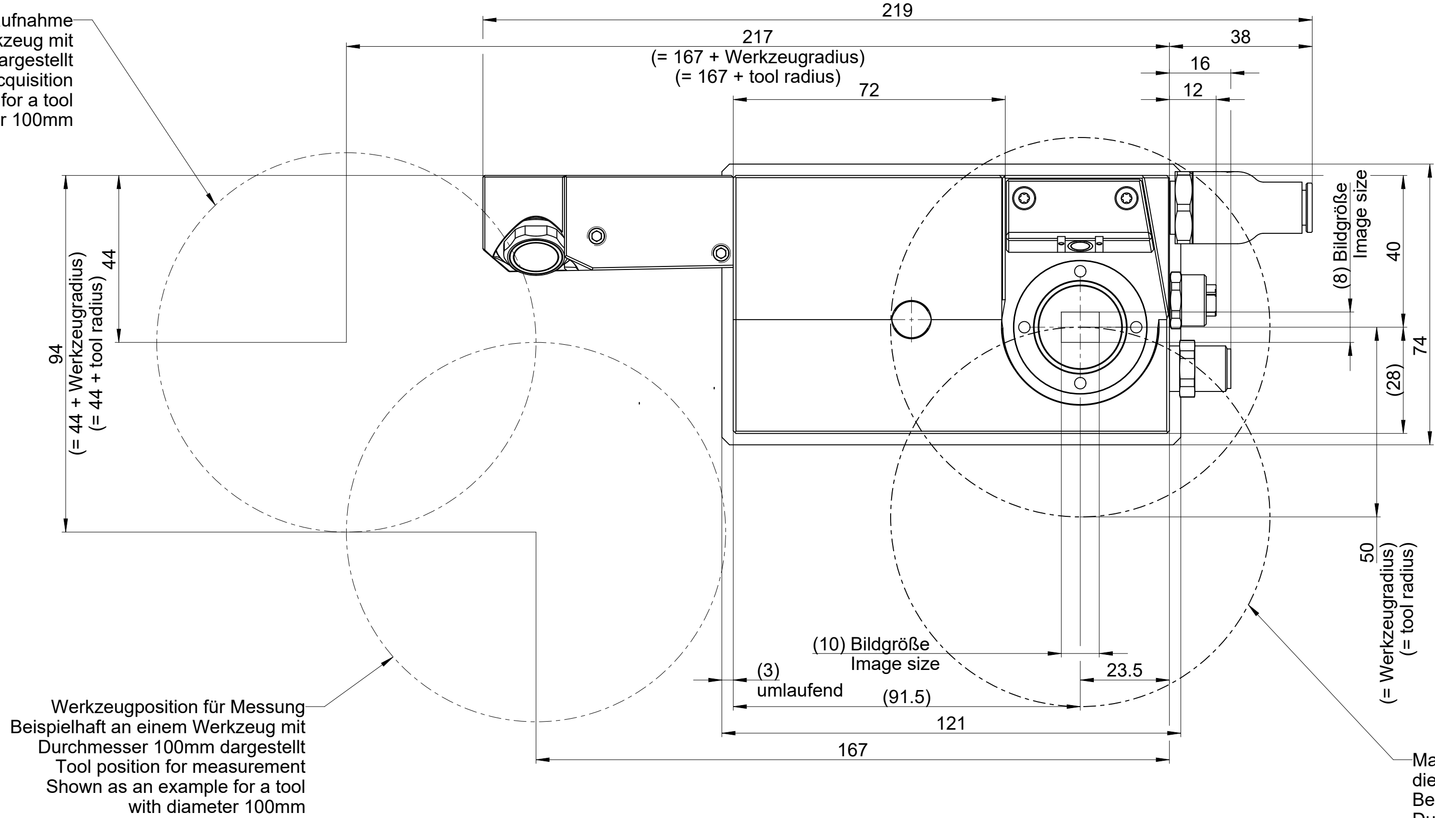
Variante 02: Ansicht ohne Zubehör Variant 02: View without accessories
