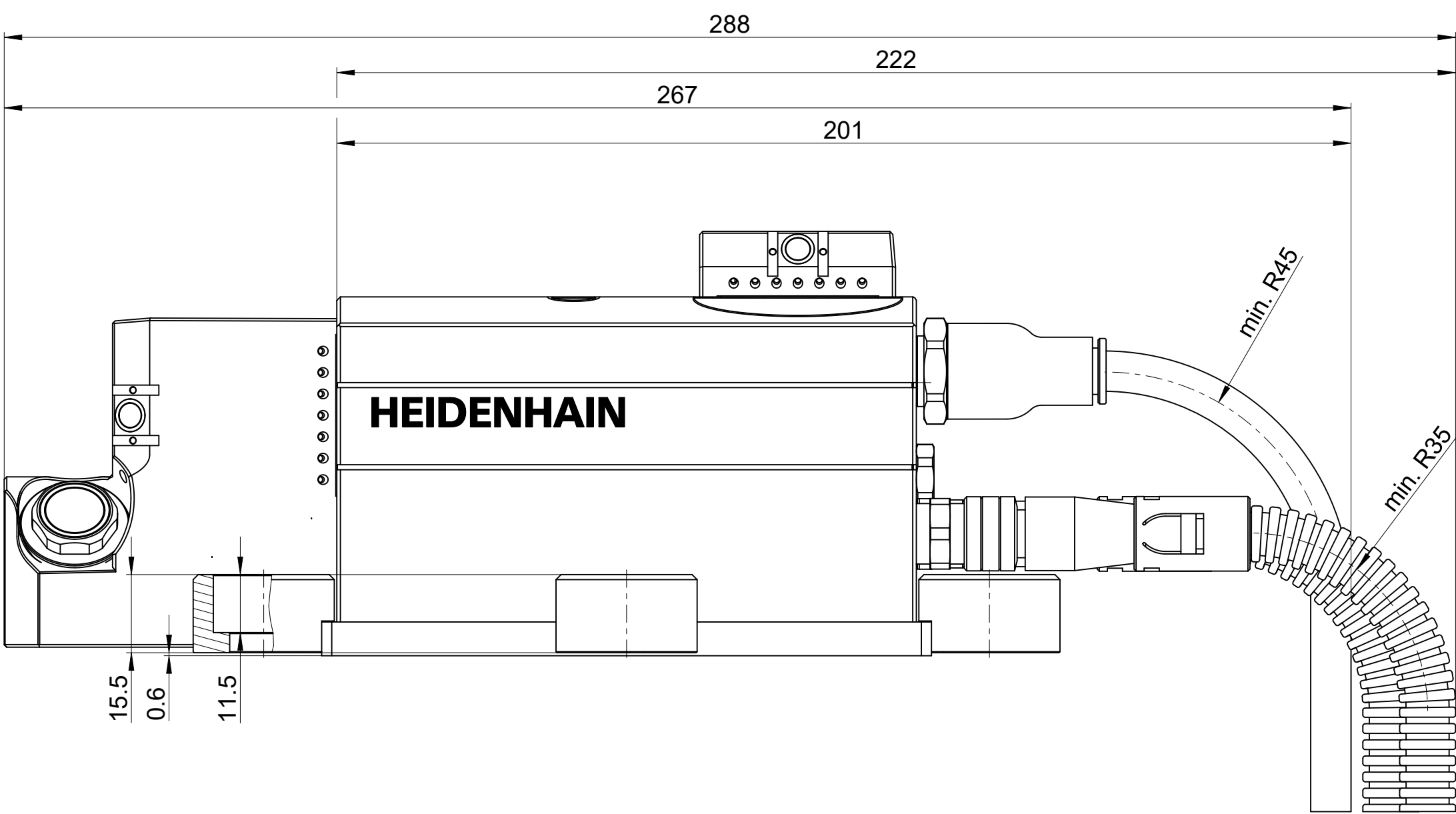
Variante 01: Ansicht mit Spannpratzen und Kabeln/Druckluftleitungen Variant 01: View with fixing clamps, cables and compressed-air tubes
