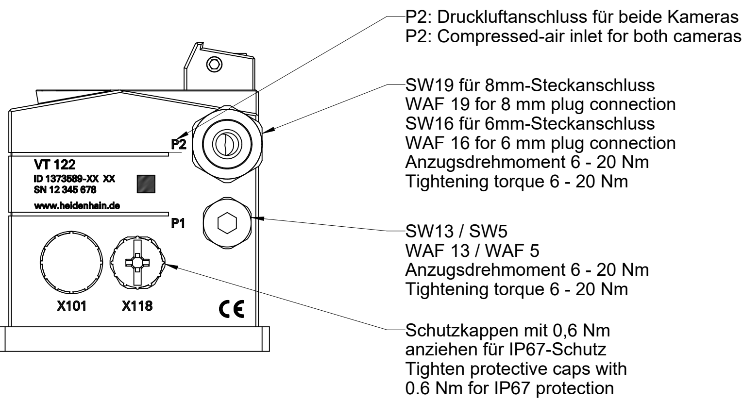
Variante 01: Ansicht mit Schutzkappen Variant 01: View with protective caps
