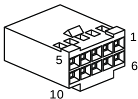
Sicht auf die Buchsenseite
