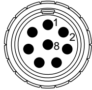
Sicht auf die Stiftseite
