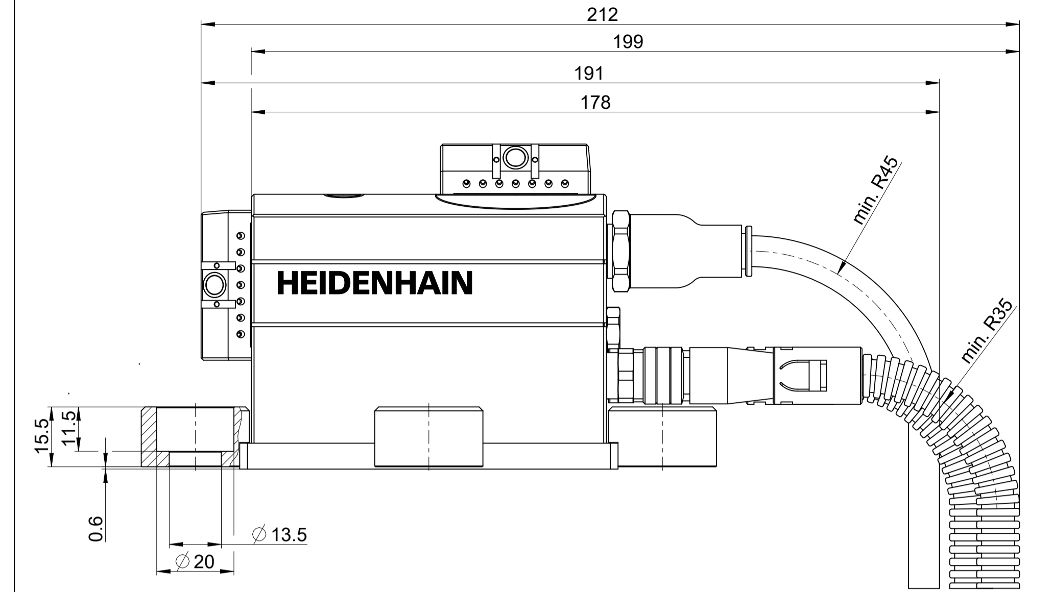
Ansicht mit Spannpratzen und Kabeln/Druckluftleitungen View with fixing clamps, cables, and compressed-air tubes
