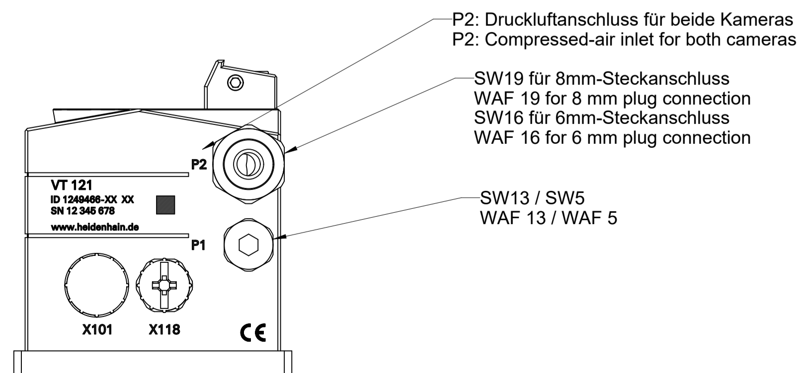
Ansicht mit Schutzkappen View with protective caps
