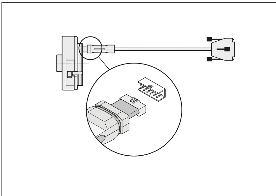
Câble de contrôle pour capteurs rotatifs encastrables
