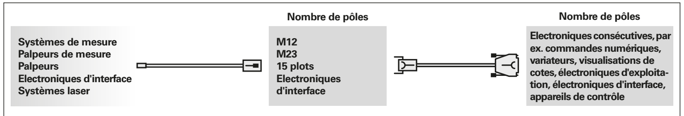
Représentation schématique des câblages
