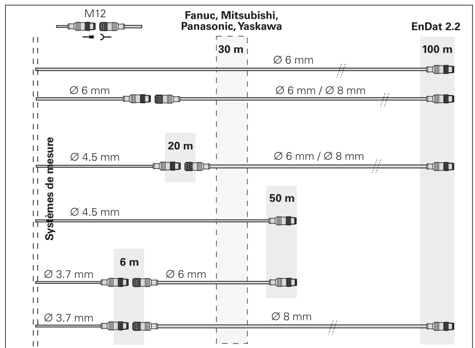
Figure 1 : Longueurs de câbles pour les interfaces série pure
