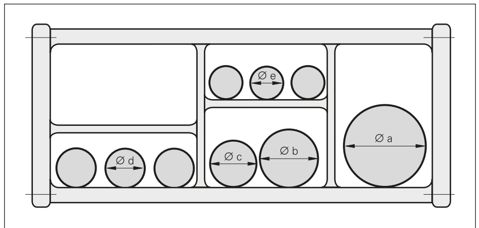
Répartition d'une chaîne porte-câbles avec différents diamètres de câbles ( \varnothing x )
