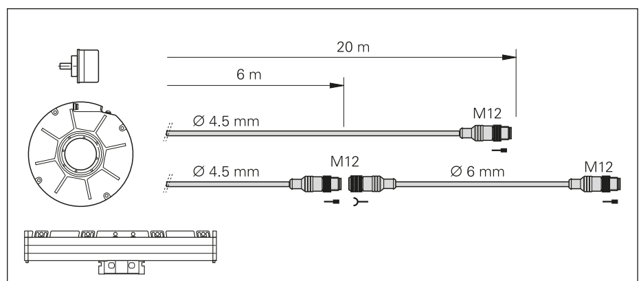
Figure 2 : Longueurs des câbles de la catégorie "Ne pas utiliser pour de nouvelles applications"
