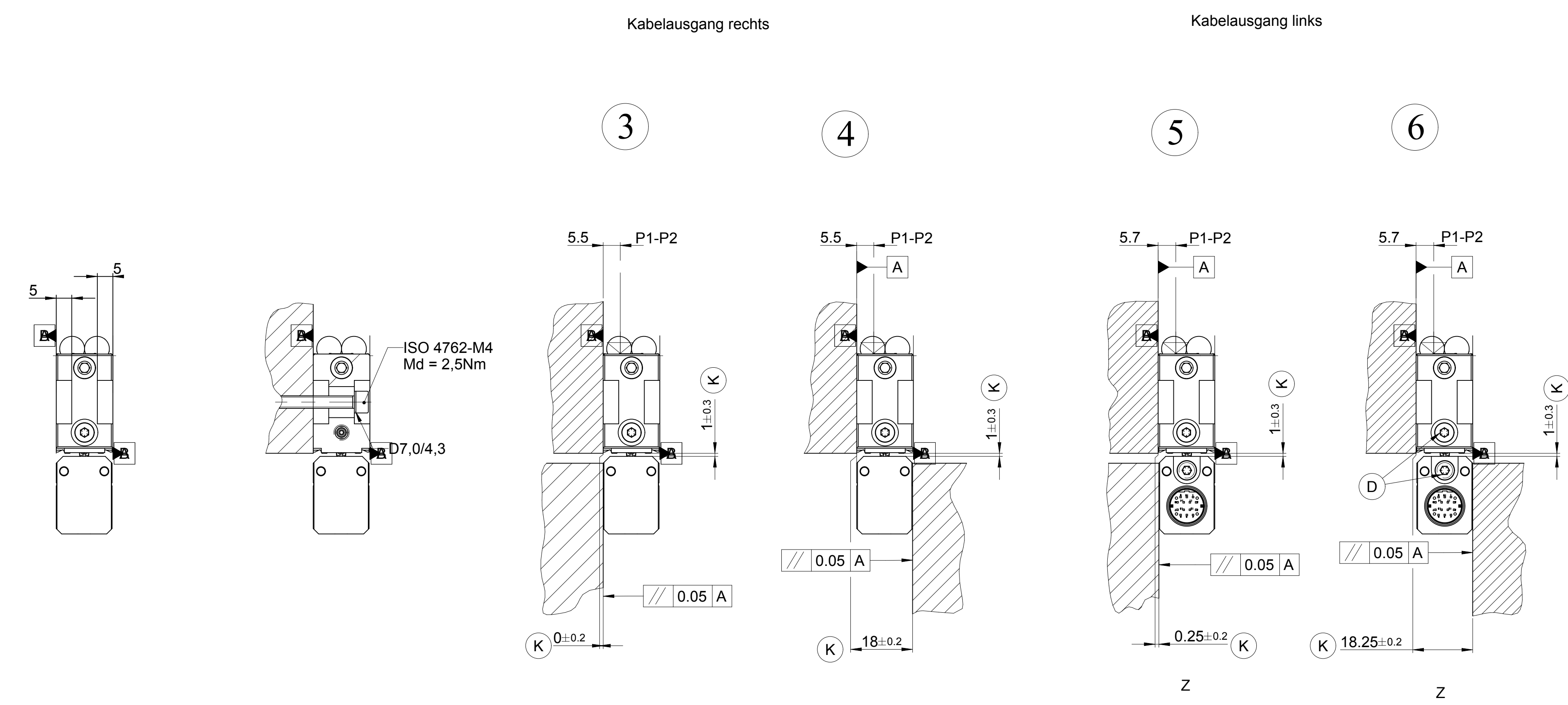
Montagemöglichkeiten mit Befestigungsendstück für M4 / Mounting possibilities with mounting block for M4
