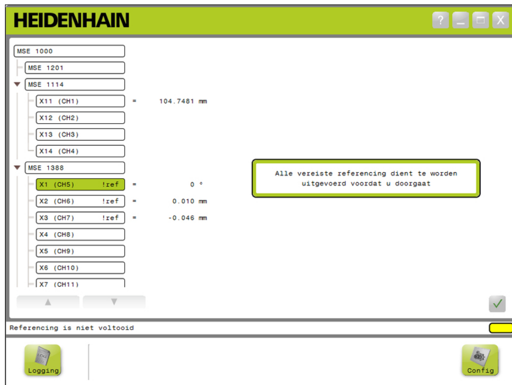
Scherm Referentieprocedure
