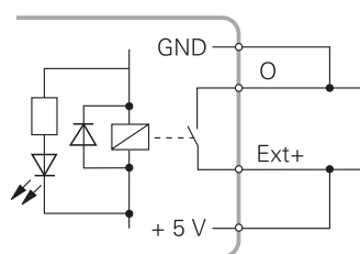
Interne DC 5 V
