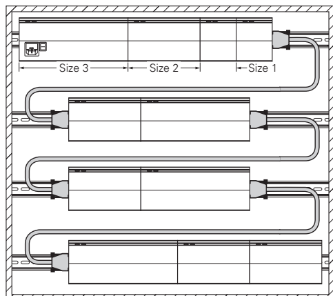
19" montagekast
