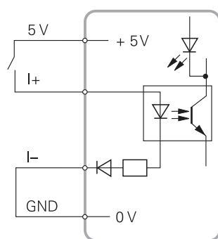
Interne DC 5 V
