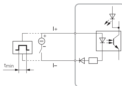
Externe voeding
