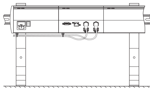
Supporto di montaggio
