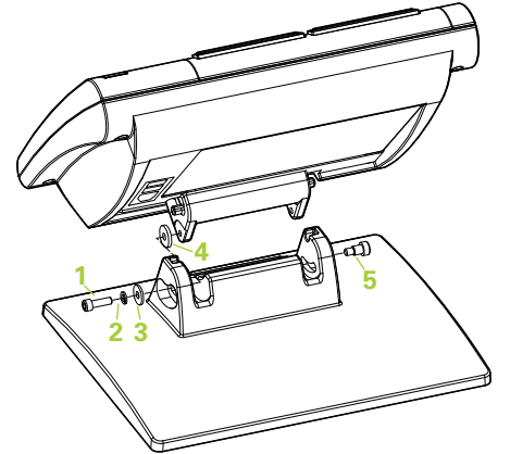
Stand kurulumu
