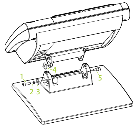
立架組合
