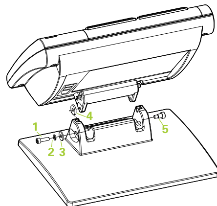
支架组件
