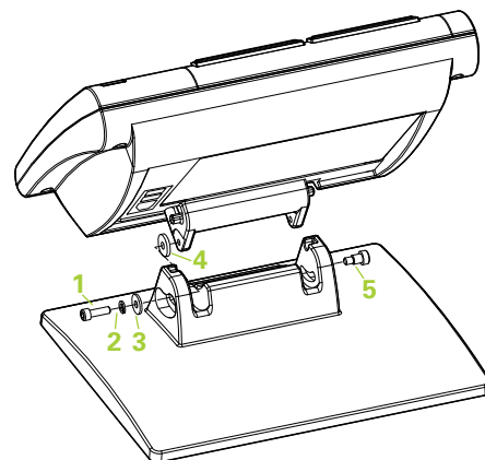
Zusammenbau des Montagefußes
