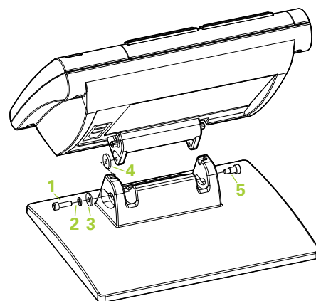
Montagevoet
