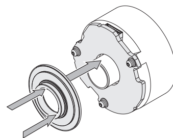
Teilkreis mit Nabe aufpressen (Messgerät A)
