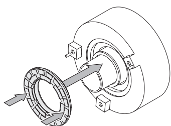
Teilkreis mit Nabe aufpressen (Messgerät B)
