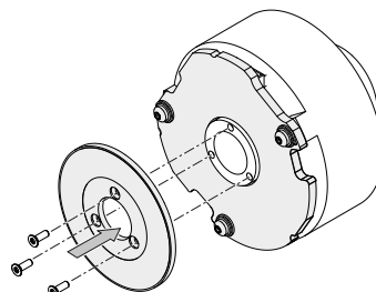
Teilkreis anschrauben (Messgerät A)
